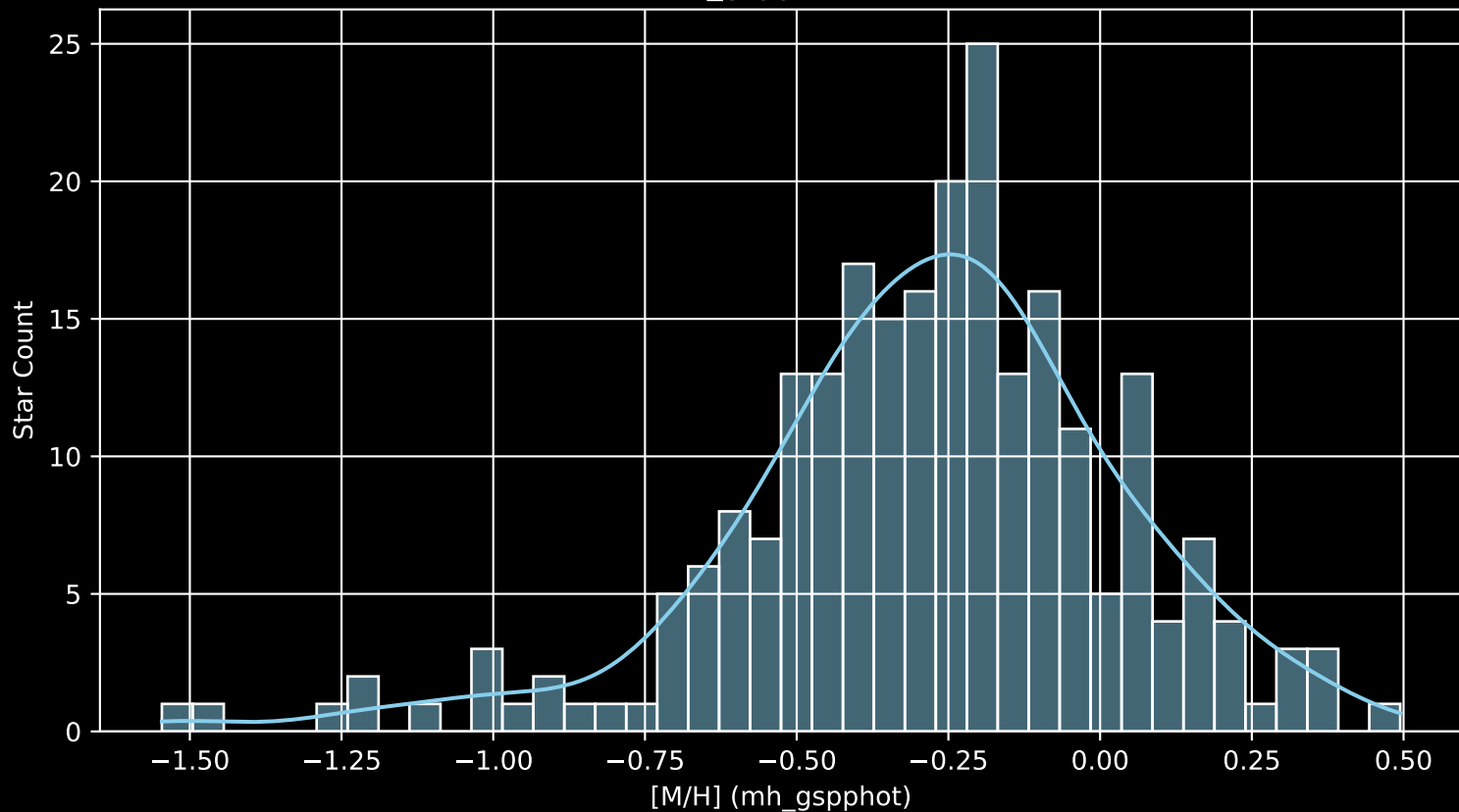
GALAH DR4 Field: [7161] [M/H] (mh_gspphot) (n= 241)
