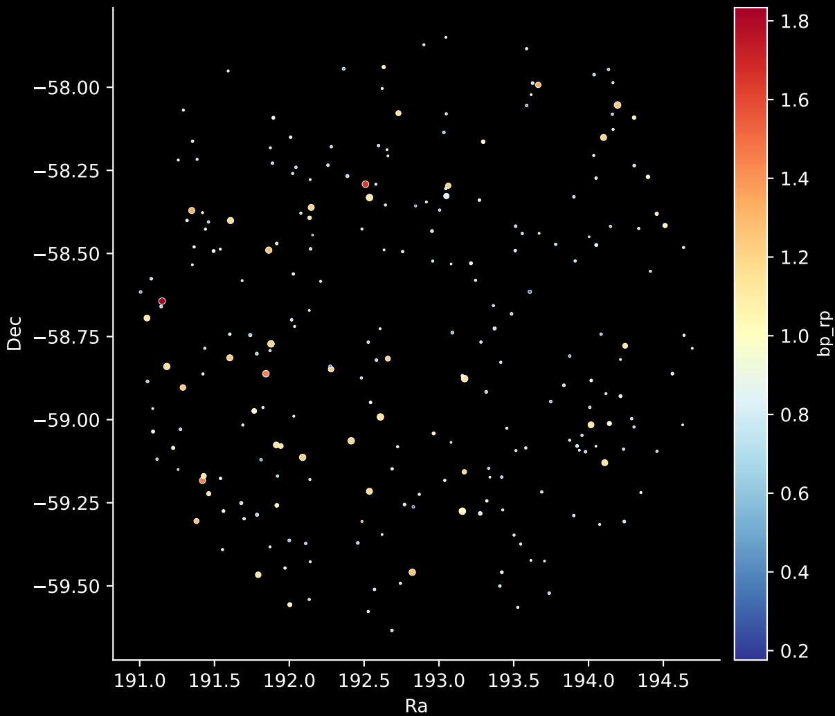
GALAH DR4 Field: [7161] Stars: 241
