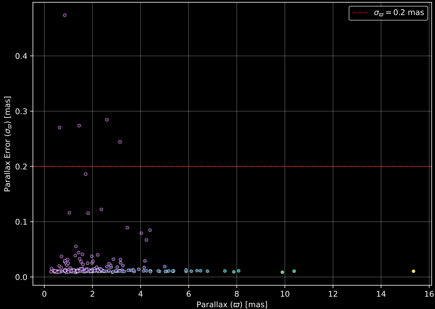
GALAH DR4 Field: [7161] Parallax Quality (n= 241)
