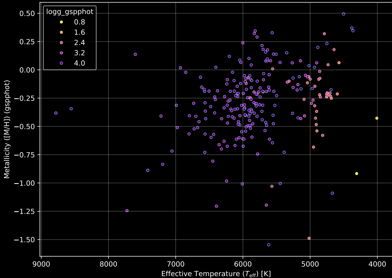
GALAH DR4 Field: [7161] Stellar Population Parameters (n= 241)
